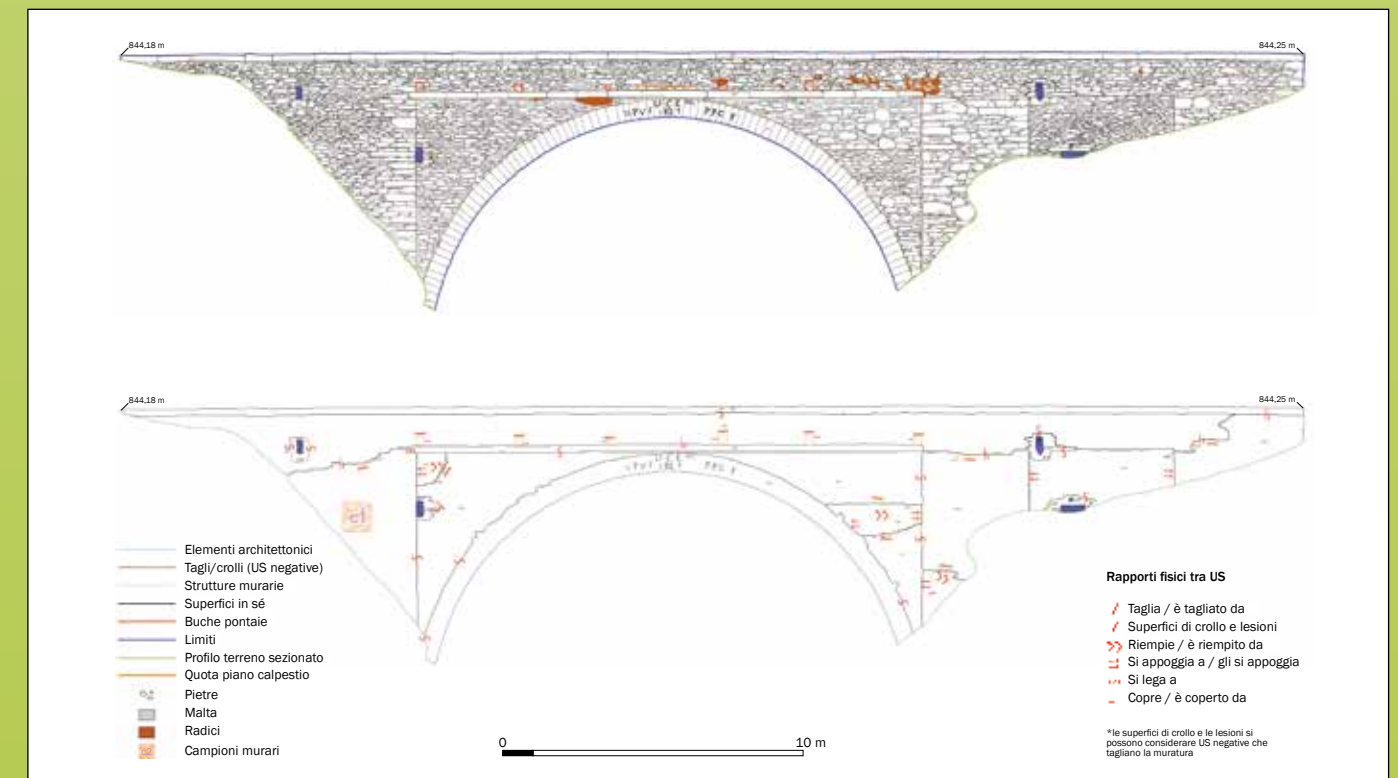
3a.-b. Il rilievo archeologico (in alto) e l'analisi stratigrafica (in basso) del prospetto sud. (Tethys Srl)
