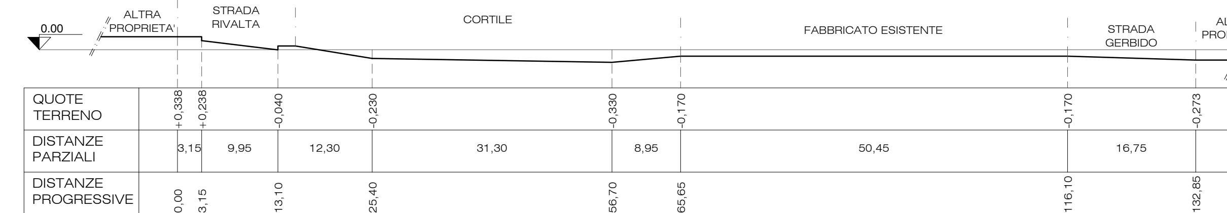
PROFILO ALTIMETRICO B-B
