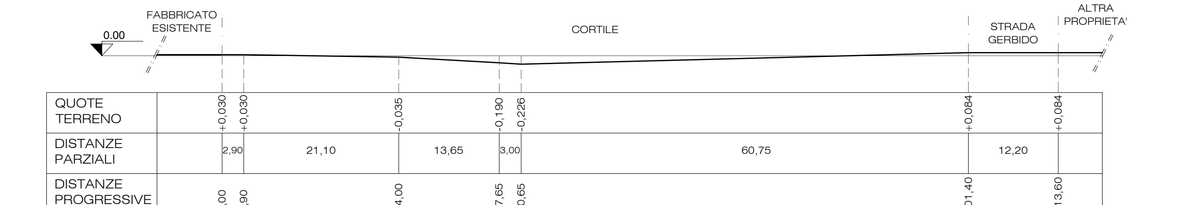
PROFILO ALTIMETRICO C-C
