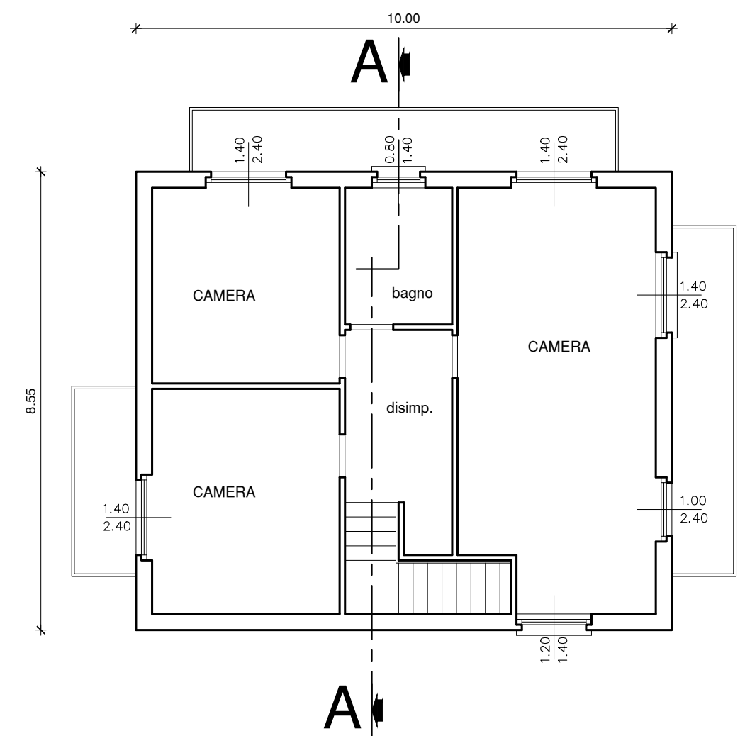
Piano primo
