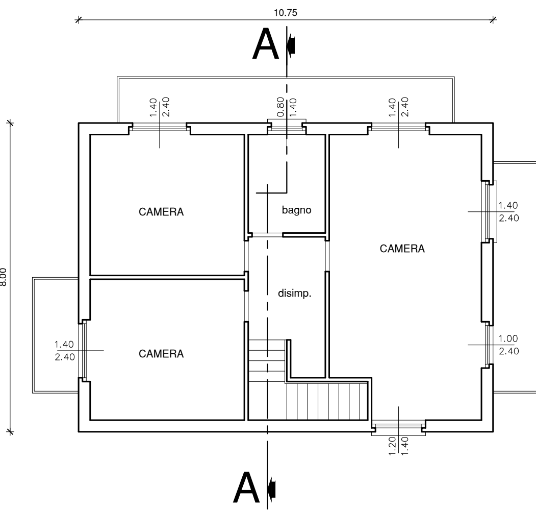
Piano primo
