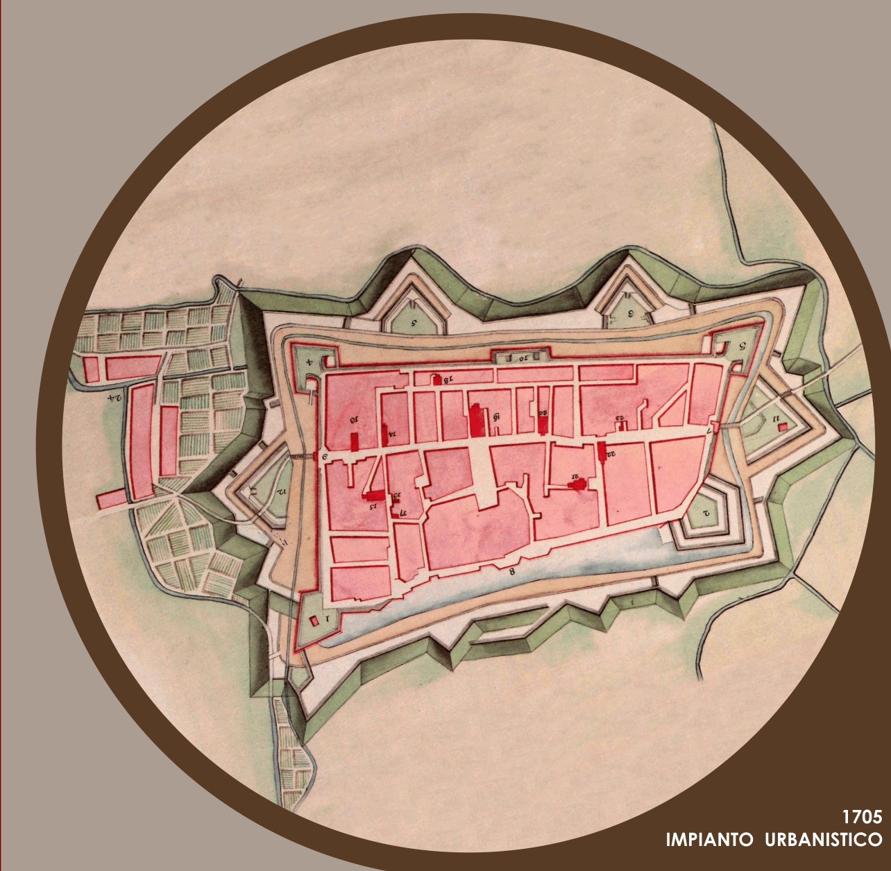
IMPIANTO URBANISTICO 1705
