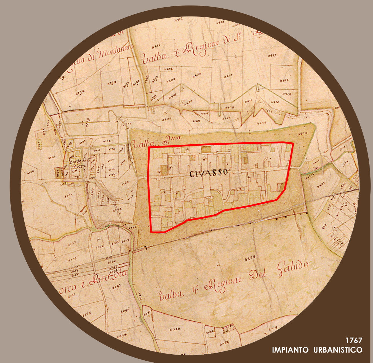
IMPIANTO URBANISTICO 1767
